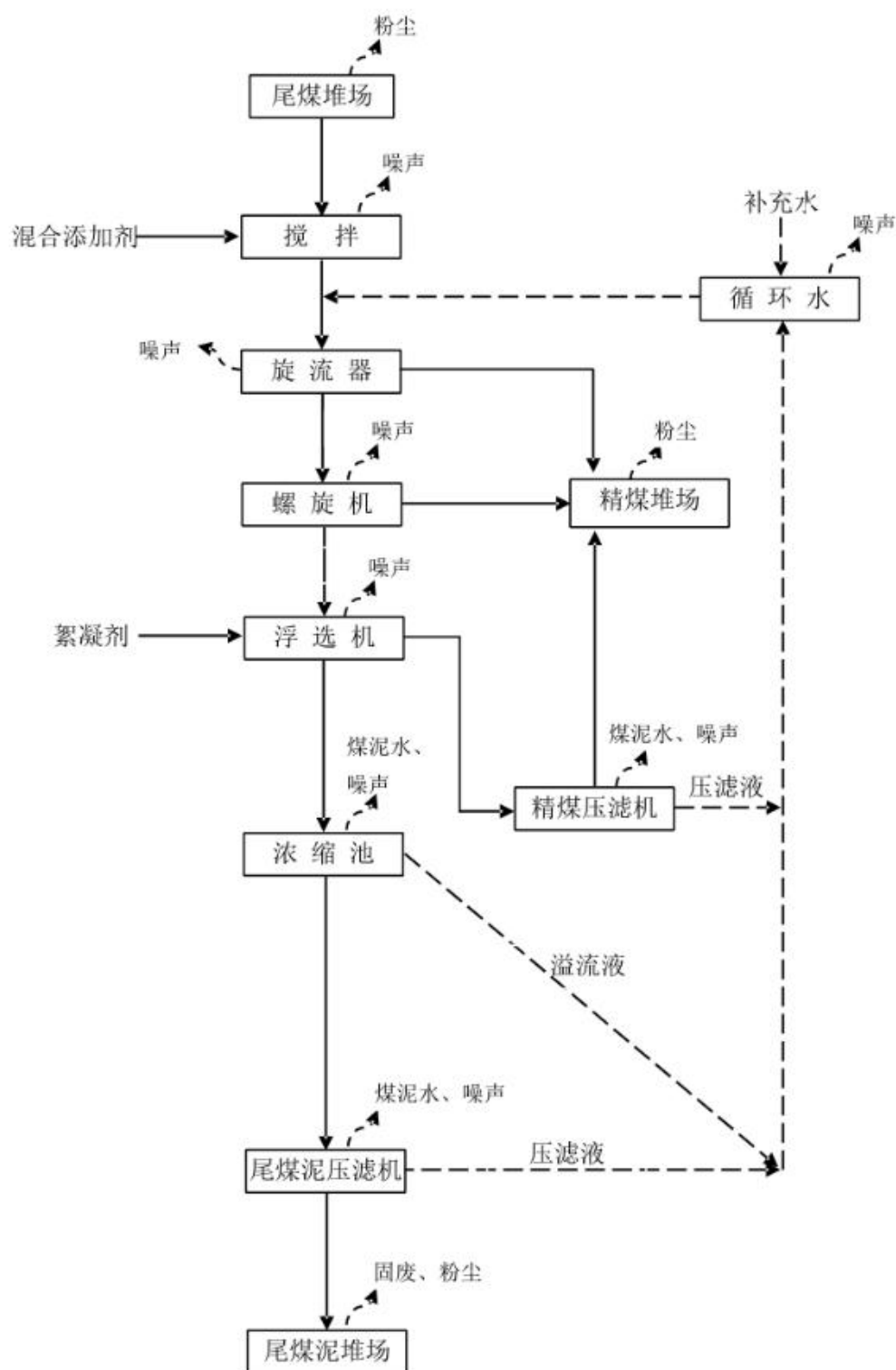
图 2-1 生产工艺流程图
