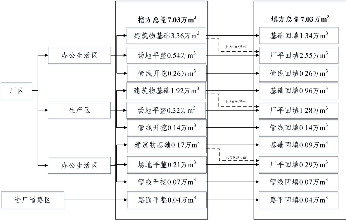
图 2-1 土石方挖填平衡图
